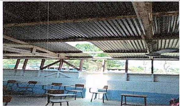
Foto 6: CAMBIO DE VIGAS POR CONSTANERAS
